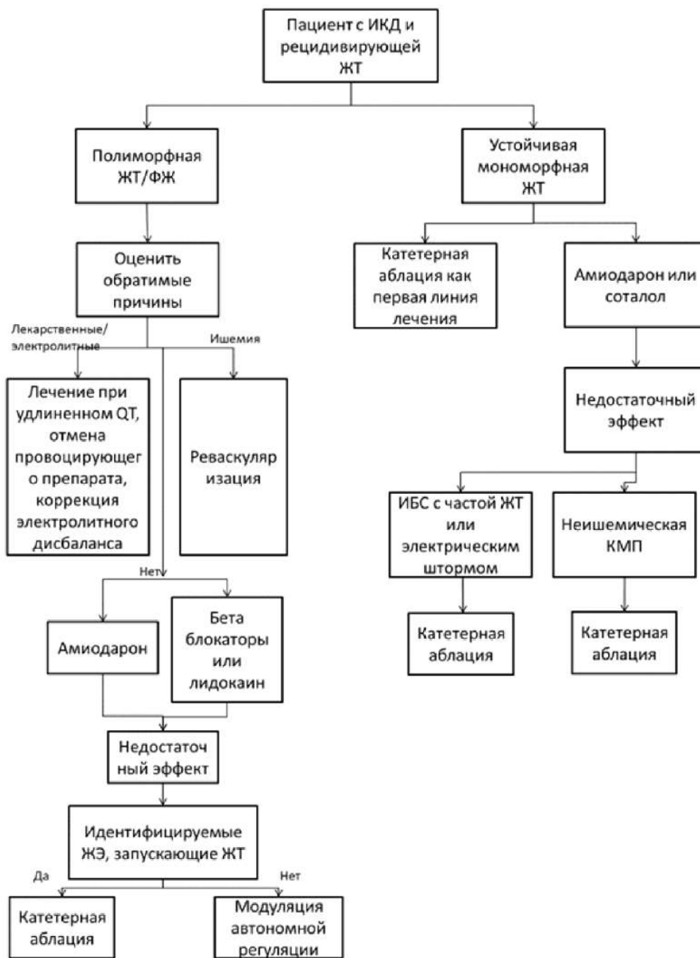
Алгоритм ведения пациента с подозрением на желудочную тахикардию
